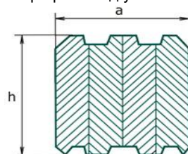
Профиль под утеплитель
