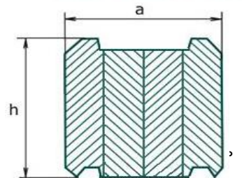
Профиль " под утеплитель"
