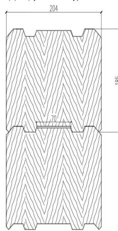
Профиль продольного пазо "без утеплителя"
