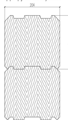
Профиль продольного пазо "без утеплителя"
