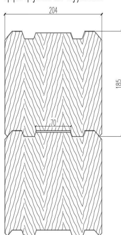
Профиль продольного пазы "без утеплителя"
