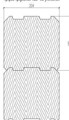
Профиль продольного пазы "без утеплителя"
